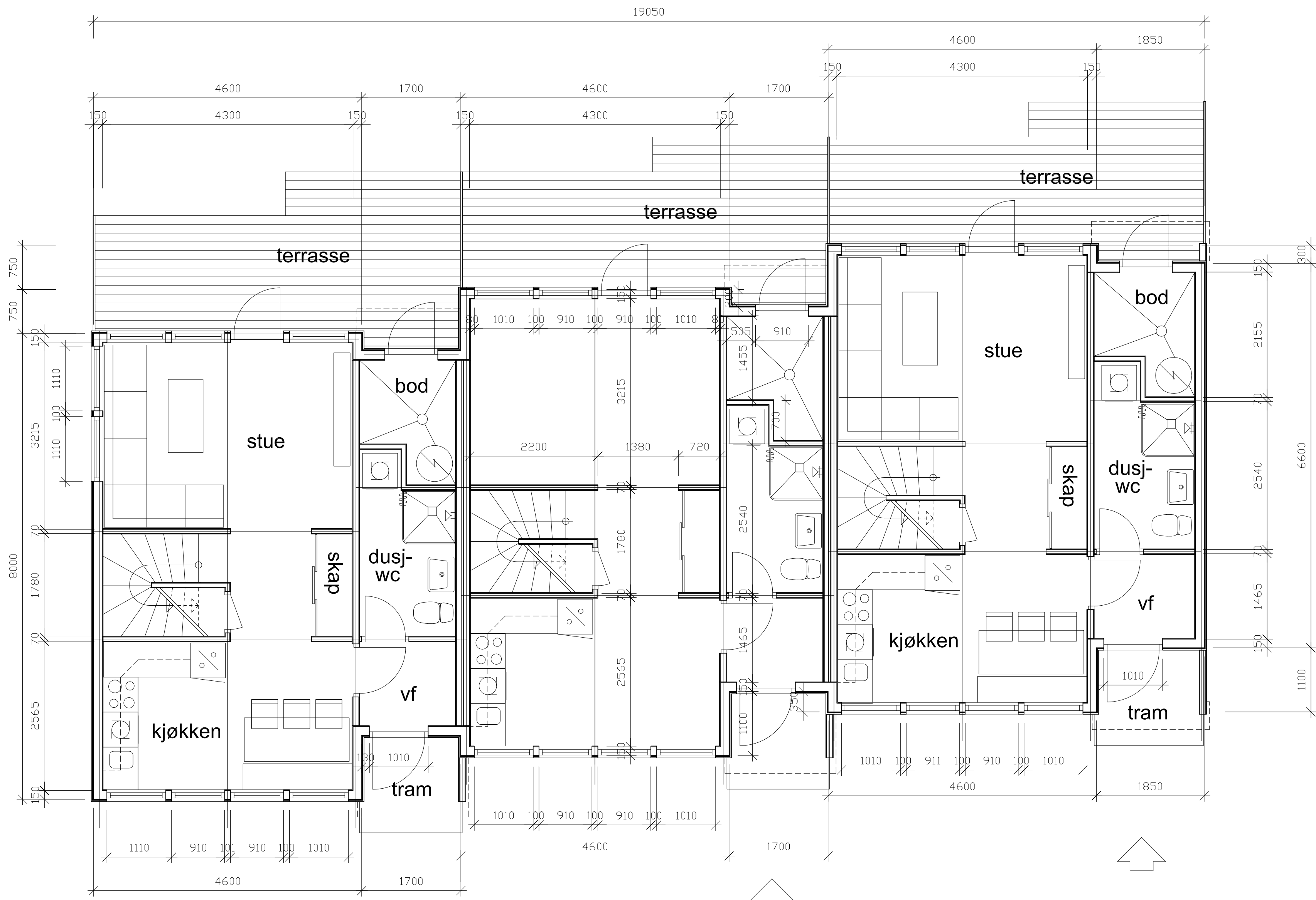
plan 1. etasje
